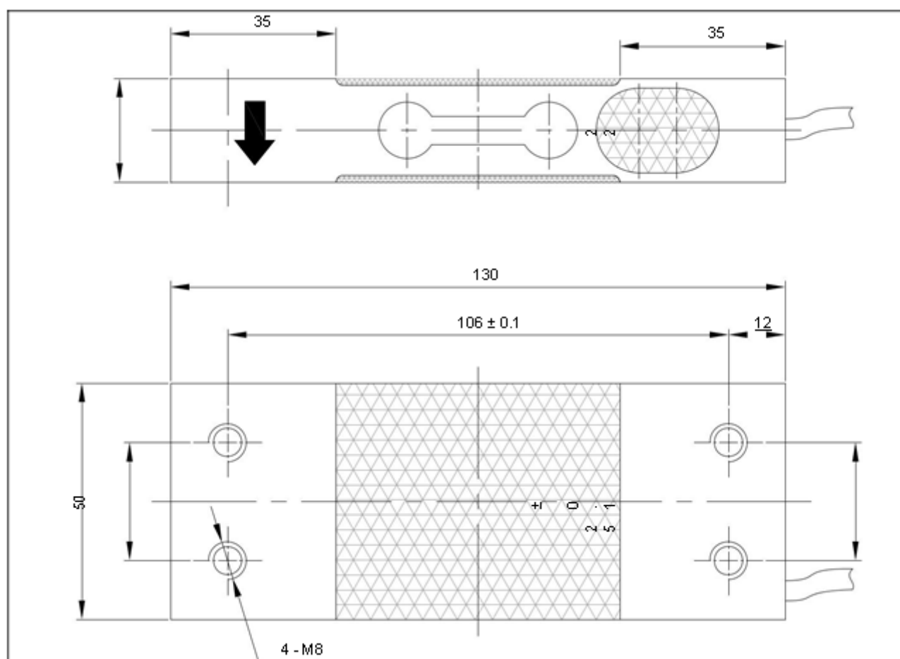
DIMENSÕES (mm)
